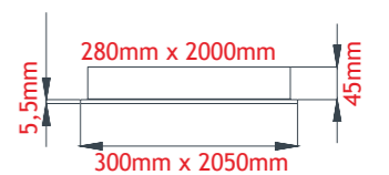
GCOP 2320
