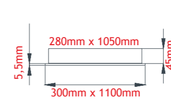
GCOP 1320 L
