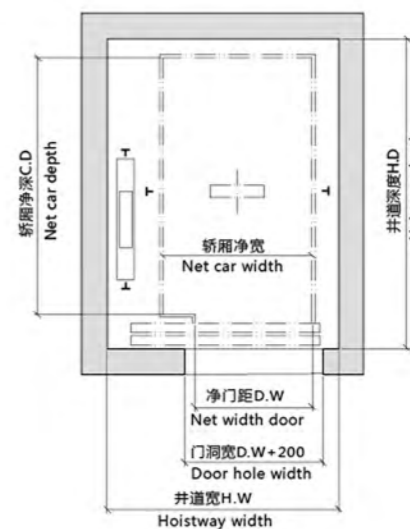
井道平面布置图 Hoistway plane layout
